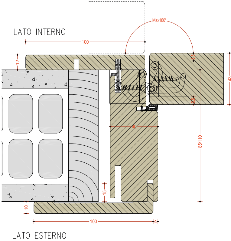
TELAIO ERA 022
