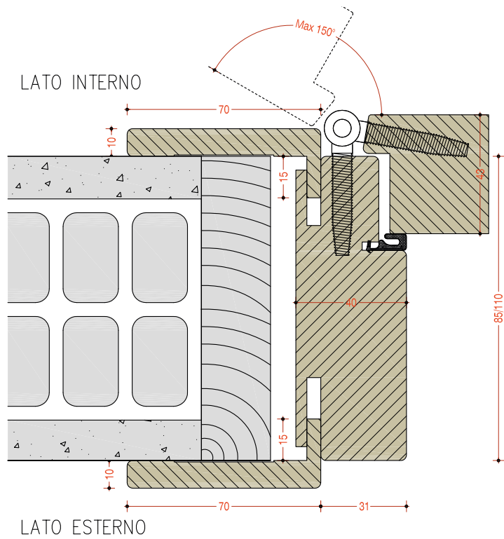
TELAIO STANDARD
